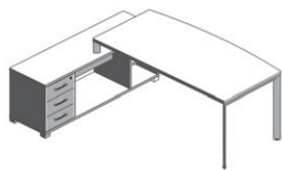
227x180xh75
